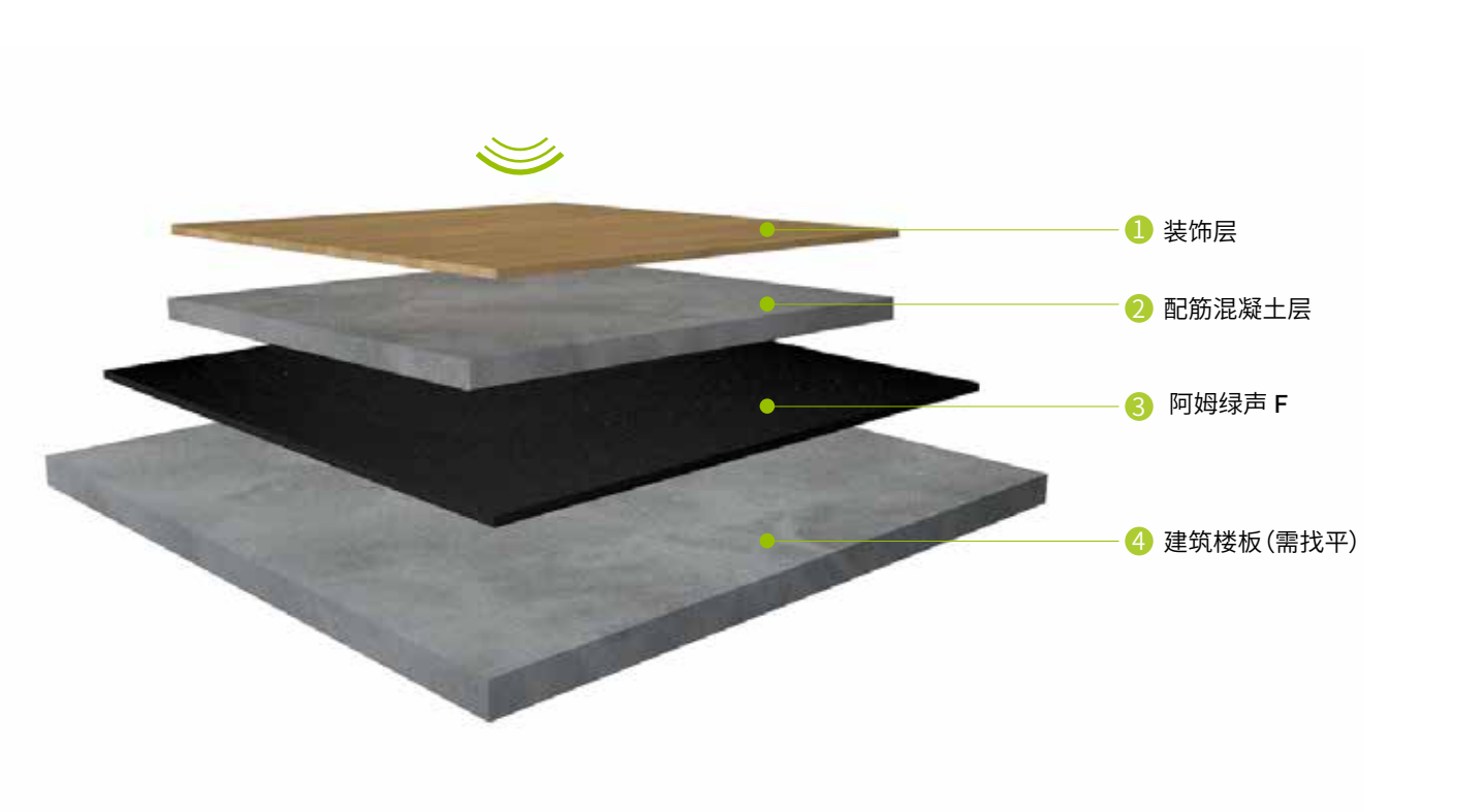
安装示意图
